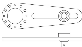
FIGUR 1 – Typisk reaktion (med glidende reaktion firkant) for PT1 til PT5
